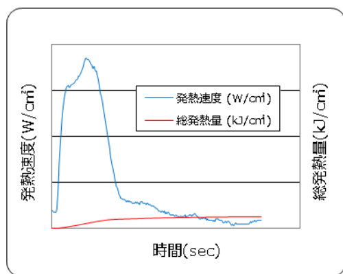
図 発熱速度と総発熱量
